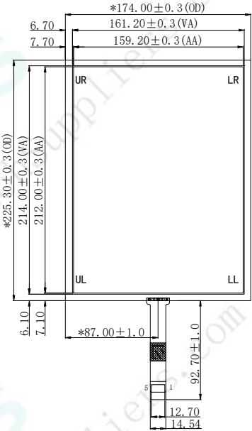
正视图
